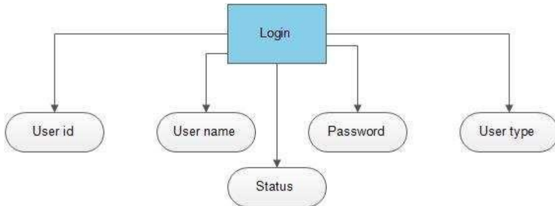
Fig 3.5: Login
